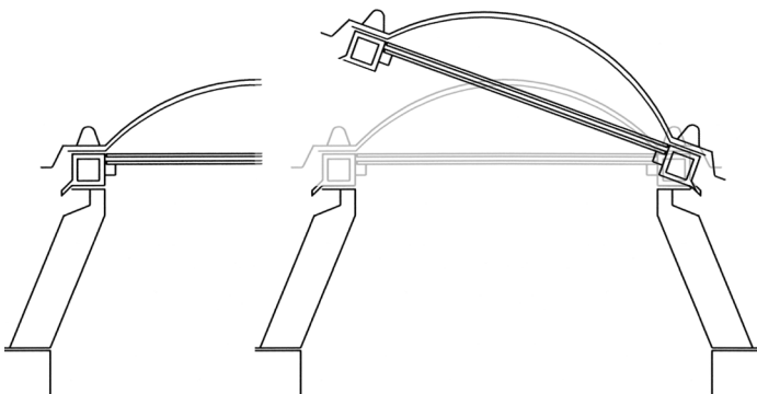
Bild 04: Die Cupolux-multiperform® ist als fix montierte Lichtkuppel und als motorisch oder manuell zu öffnende Lüftungsklappe lieferbar. Bei der letzteren sind der Rahmen mit Sicherheitsverglasung und die Lichtkuppel fest verschraubt und über Scharniere und Verschlussmechanismus mit einem Montagerahmen auf dem Aufsetzkranz verbunden. Der elektrische Antrieb ist verdeckt im Rahmen eingebaut.
