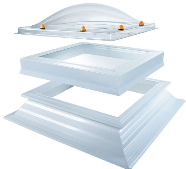
Bild 02: Die Cupolux-multiperform® Lichtkuppel besteht aus einem neuen (oder bereits vorhandenen) Aufsetzkranz, dem mittleren Rahmen mit 2-fach-Isolierverglasung und der äusseren 2-schaligen Lichtkuppel. Die Montage ist schnell und einfach. Auch bei Sanierungen sind keine aufwendigen Anpassungen erforderlich.
